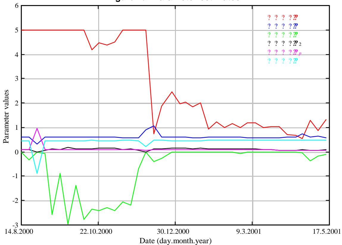
Figure 1a: Parameter estimates
